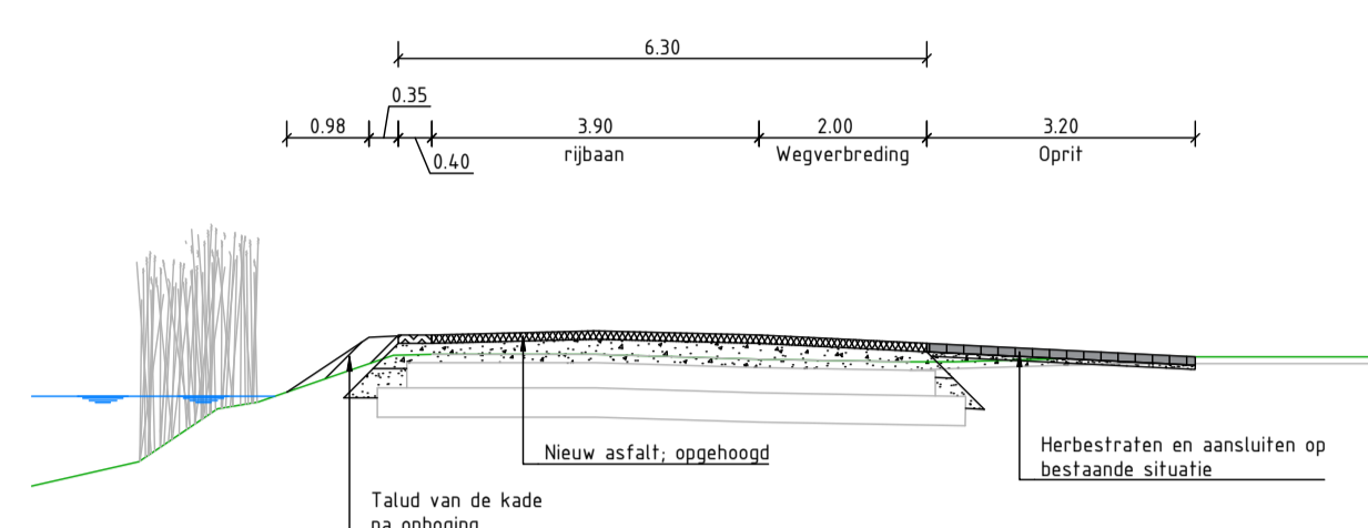
DWARSPROFIEL 2 schaal 1:100
