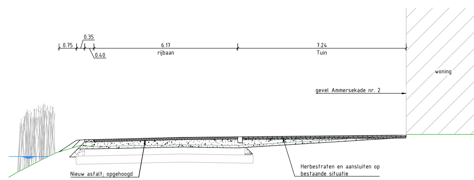
DWARSPROFIEL 4 schaal 1:100
