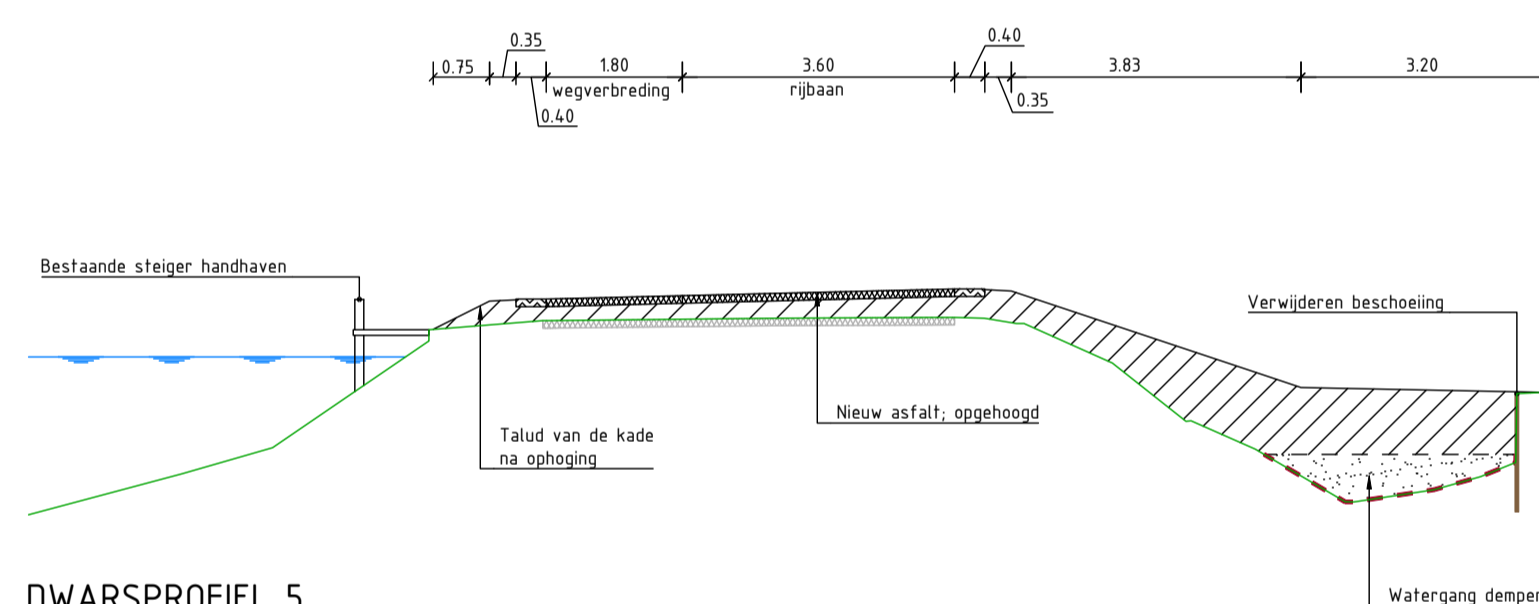
DWARSPROFIEL 5 schaal 1:100
