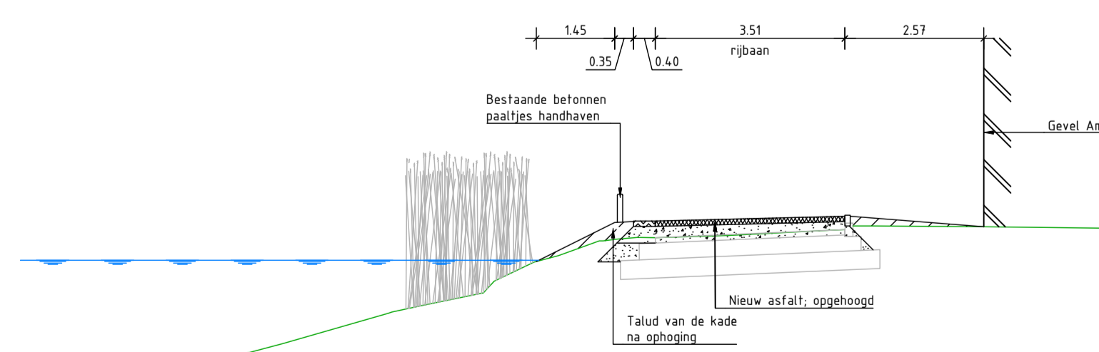
DWARSPROFIEL 7 schaal 1:100
