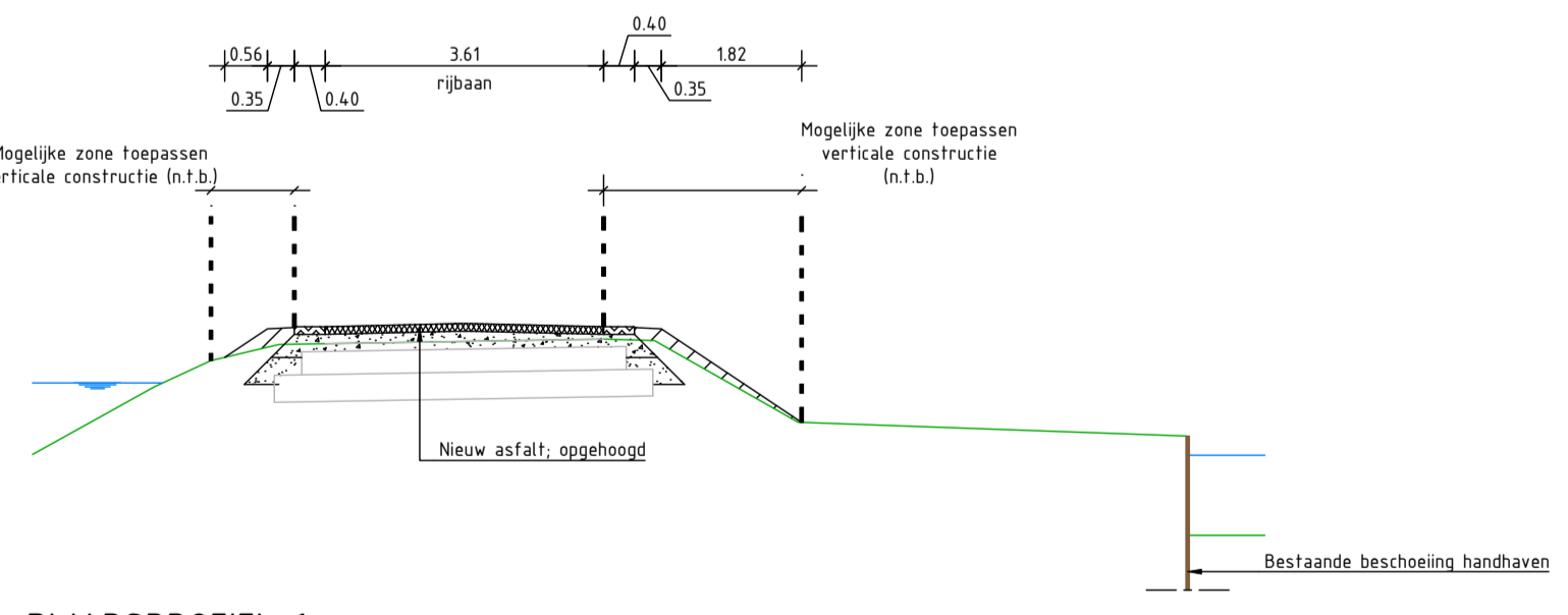
DWARSPROFIEL 6 schaal 1:100
